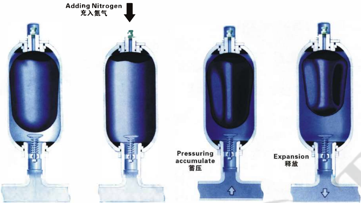
图1 Fig.1 蓄能器工作示意图
